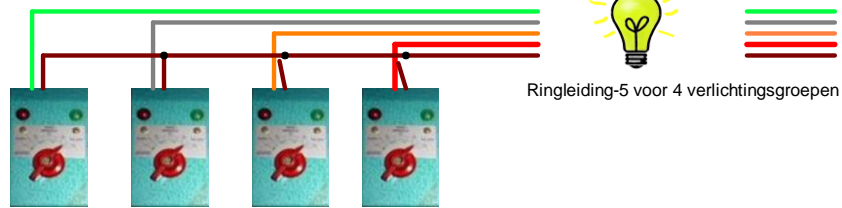
4x Trafo 50 VA Temsi 202
